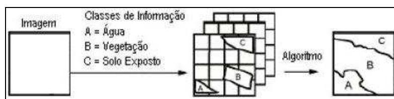
Figura 56: Representação da classificação supervisionada. Fonte: Noguchi, 2004.
