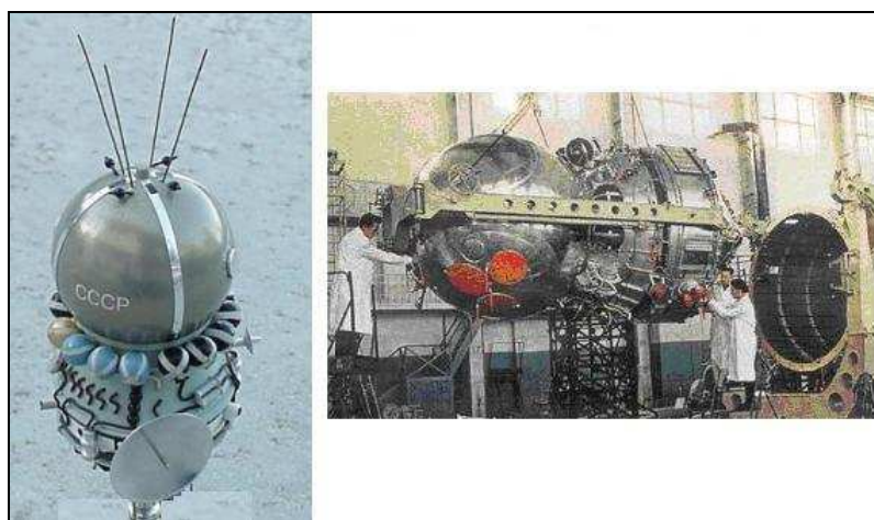
Figura 13: Satélite soviético Zenit e a preparação do foguete para o seu lançamento.
