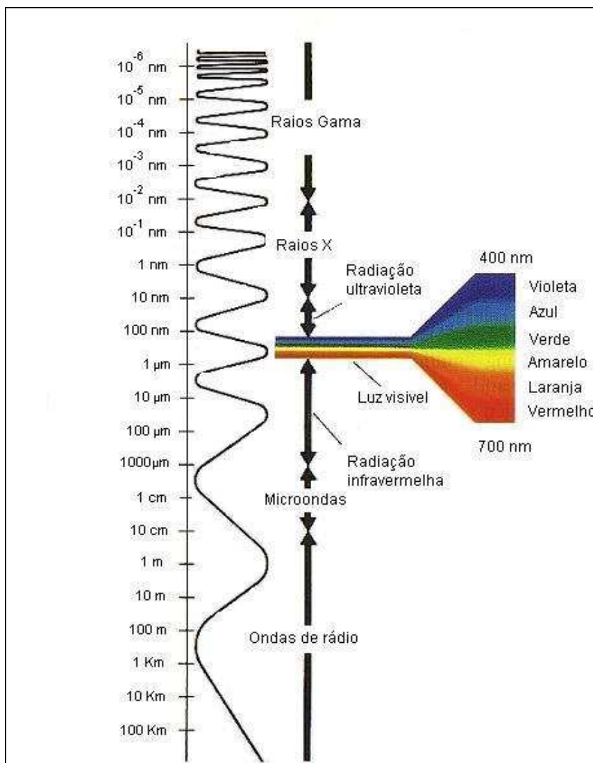
Figura 35: Espectro eletromagnético.
