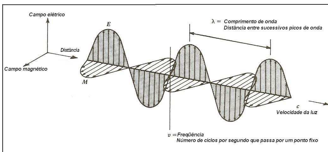
Figura 33: Onda eletromagnética. Fonte: Adaptado de Lillesand et al , 2004 (p.4)
