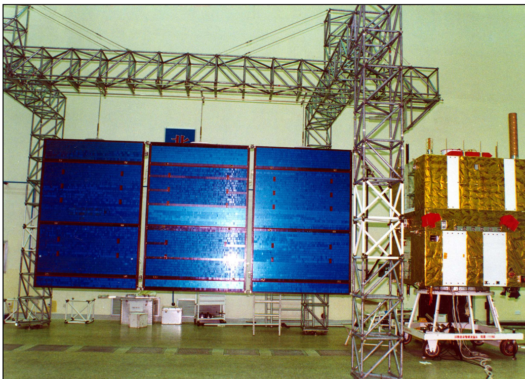
Figura 26: Satélite CBERS-I.
