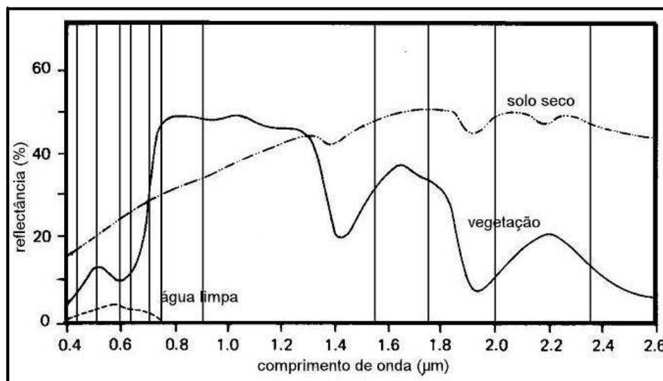
Figura 37: Assinatura espectral. Fonte: Adaptado de Lillesand et al , 2004 (p.17).
