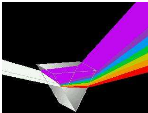
Figura 34: Decomposição da luz solar no prisma
