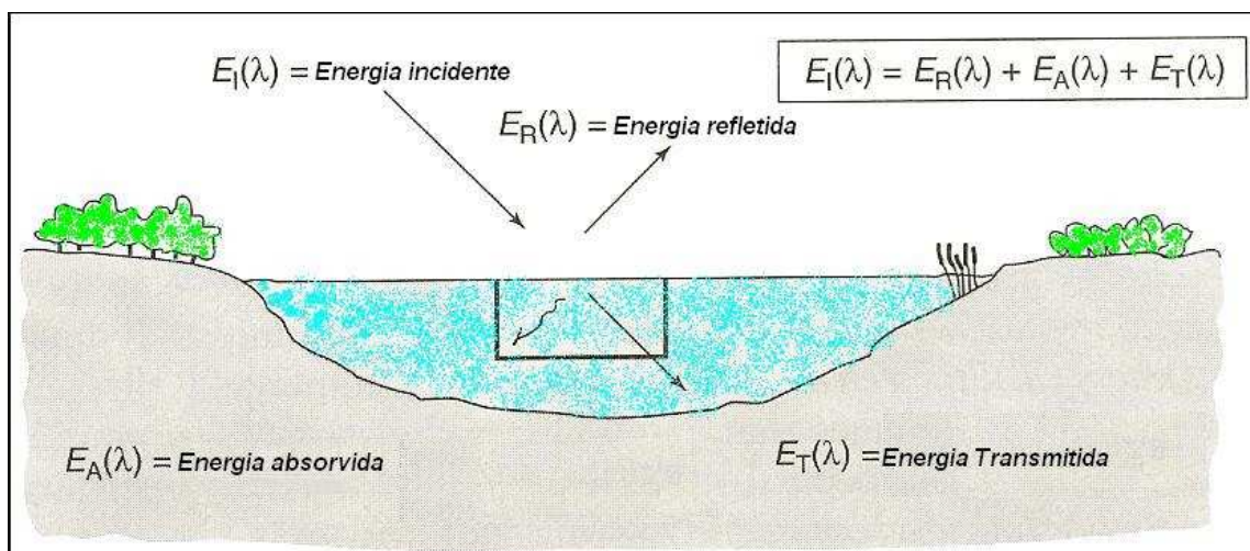
Figura 36: Interação entre a energia eletromagnética e as feições da Terra. Fonte: Adaptado de Lillesand et al , 2004 (p.12).
