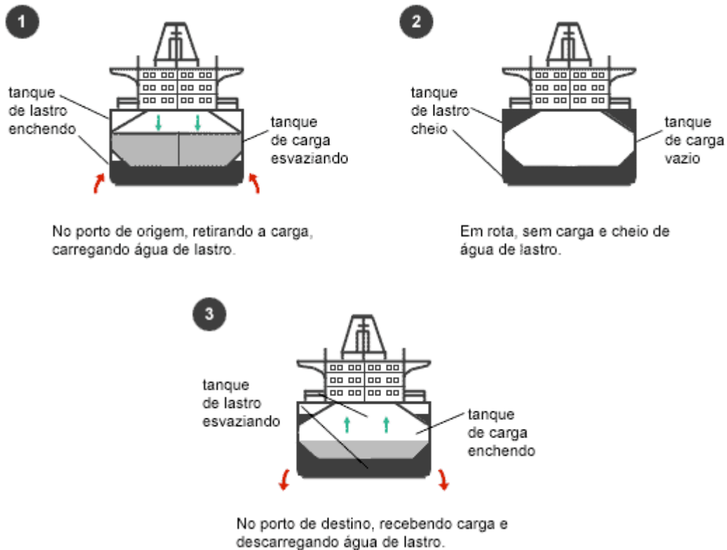
Vista em corte do navio cargueiro
